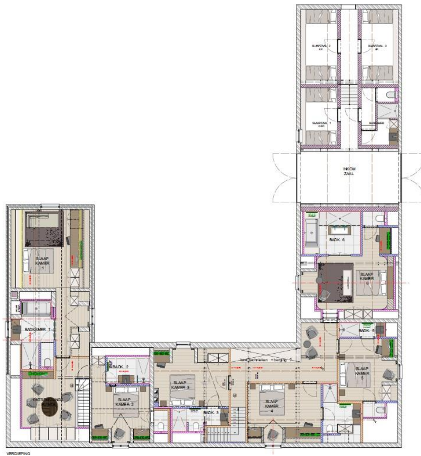
Plan bovenverdieping
